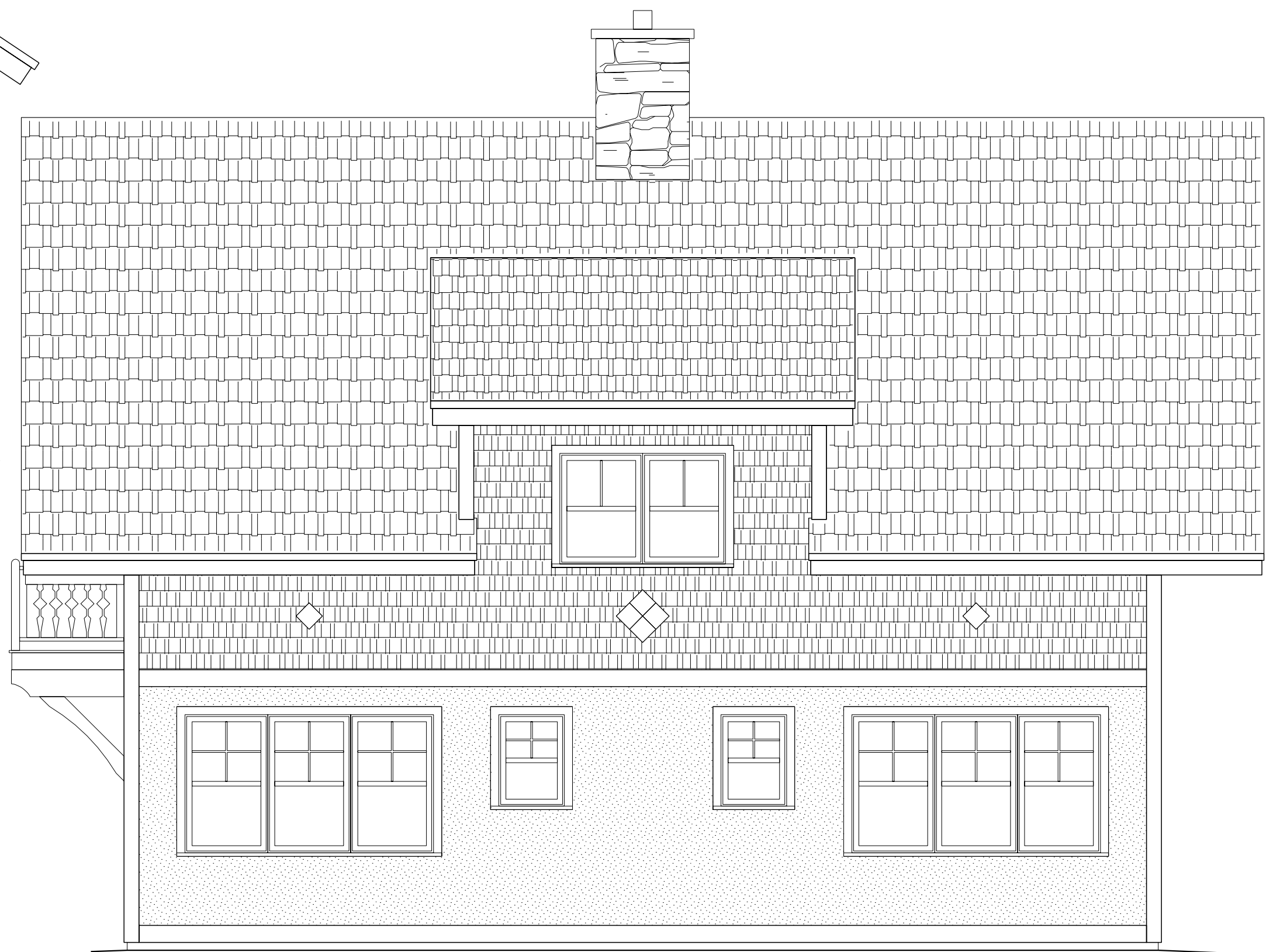
2 RIGHT ELEVATION
